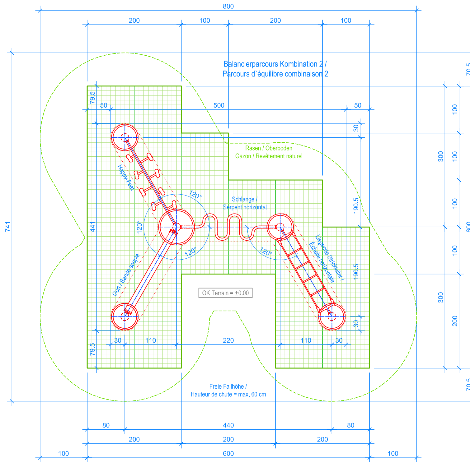
GRUNDRISS / PLAN 1:50
