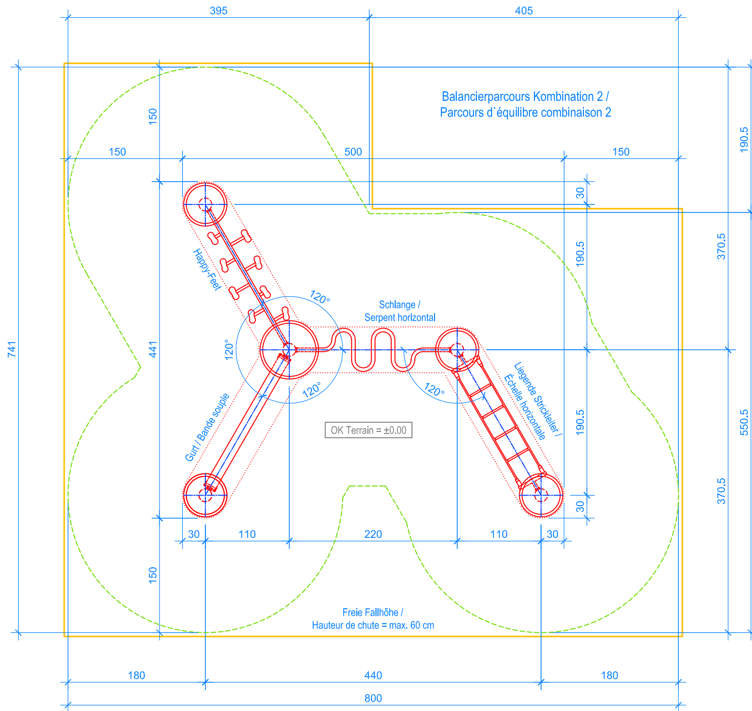
GRUNDRISS / PLAN 1:50
