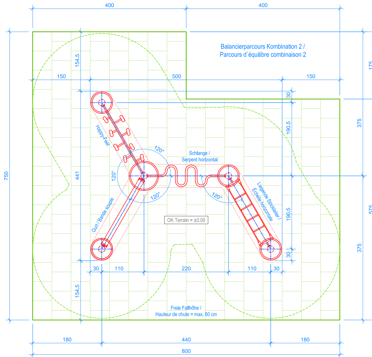
GRUNDRISS / PLAN 1:50
