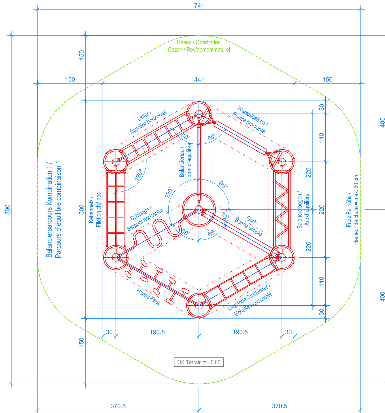
GRUNDRISS / PLAN 1:50
