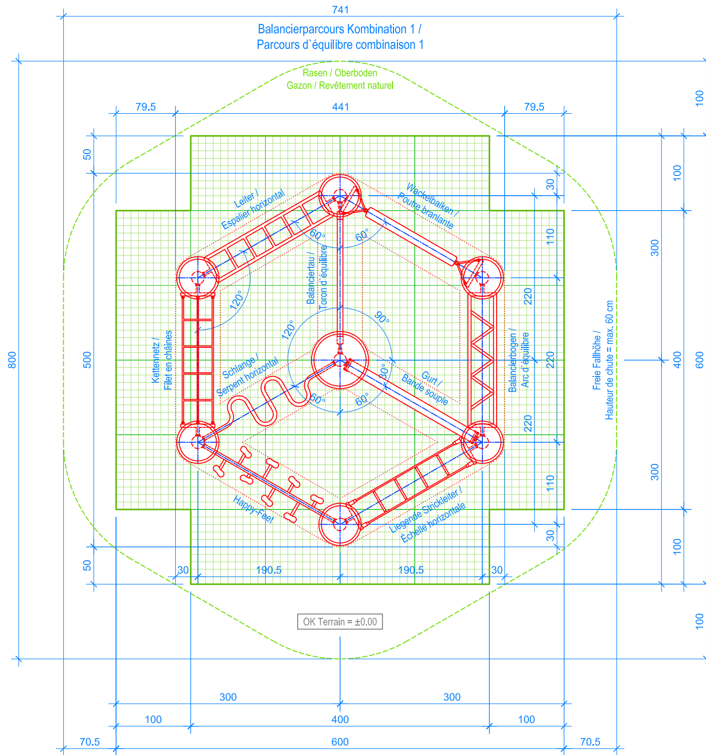
GRUNDRISS / PLAN 1:50
