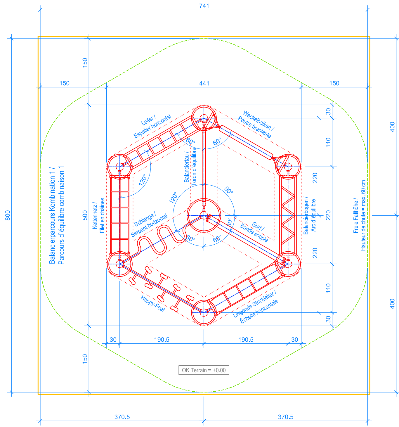
GRUNDRISS / PLAN 1:50
