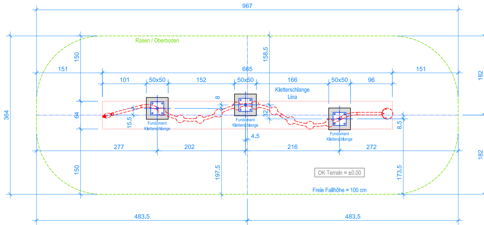
GRUNDRISS 1:50
