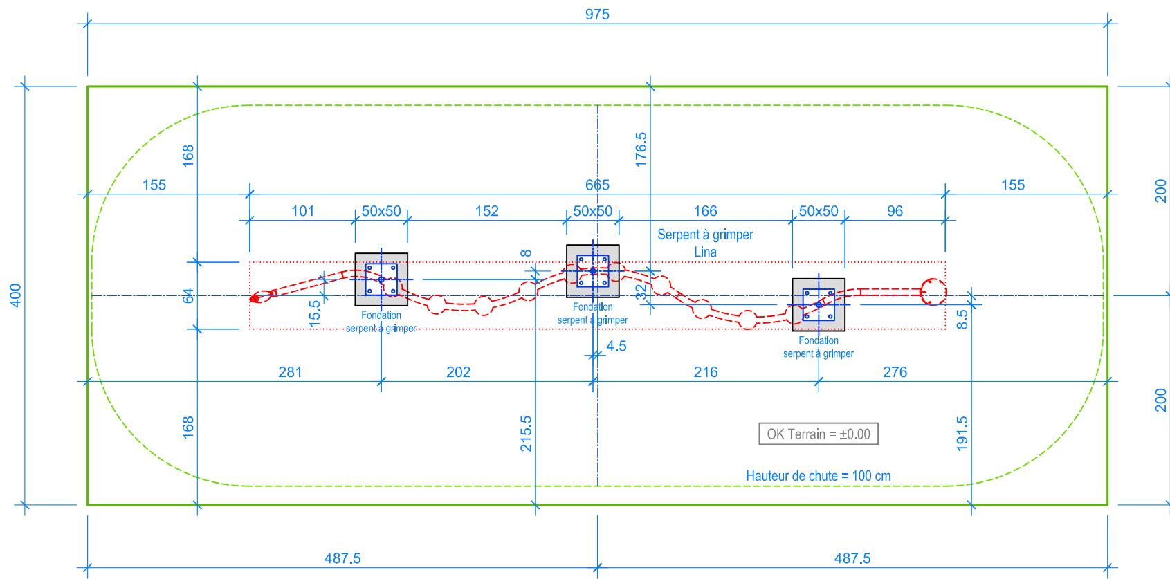
PLAN 1:50
