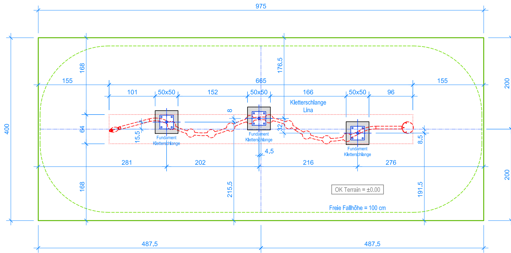
GRUNDRISS 1:50
