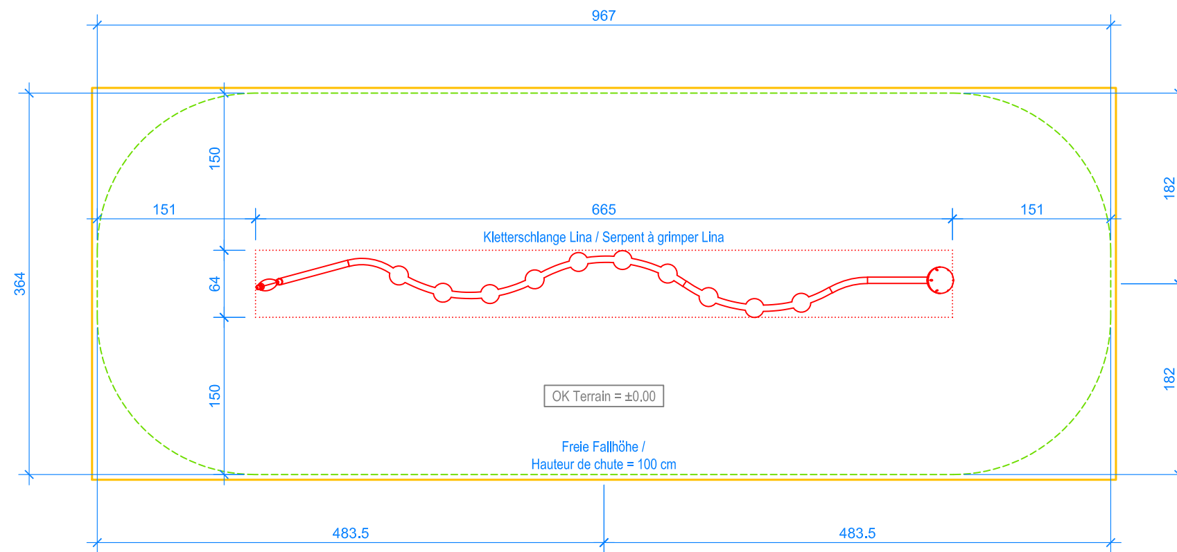
GRUNDRISS / PLAN 1:50
