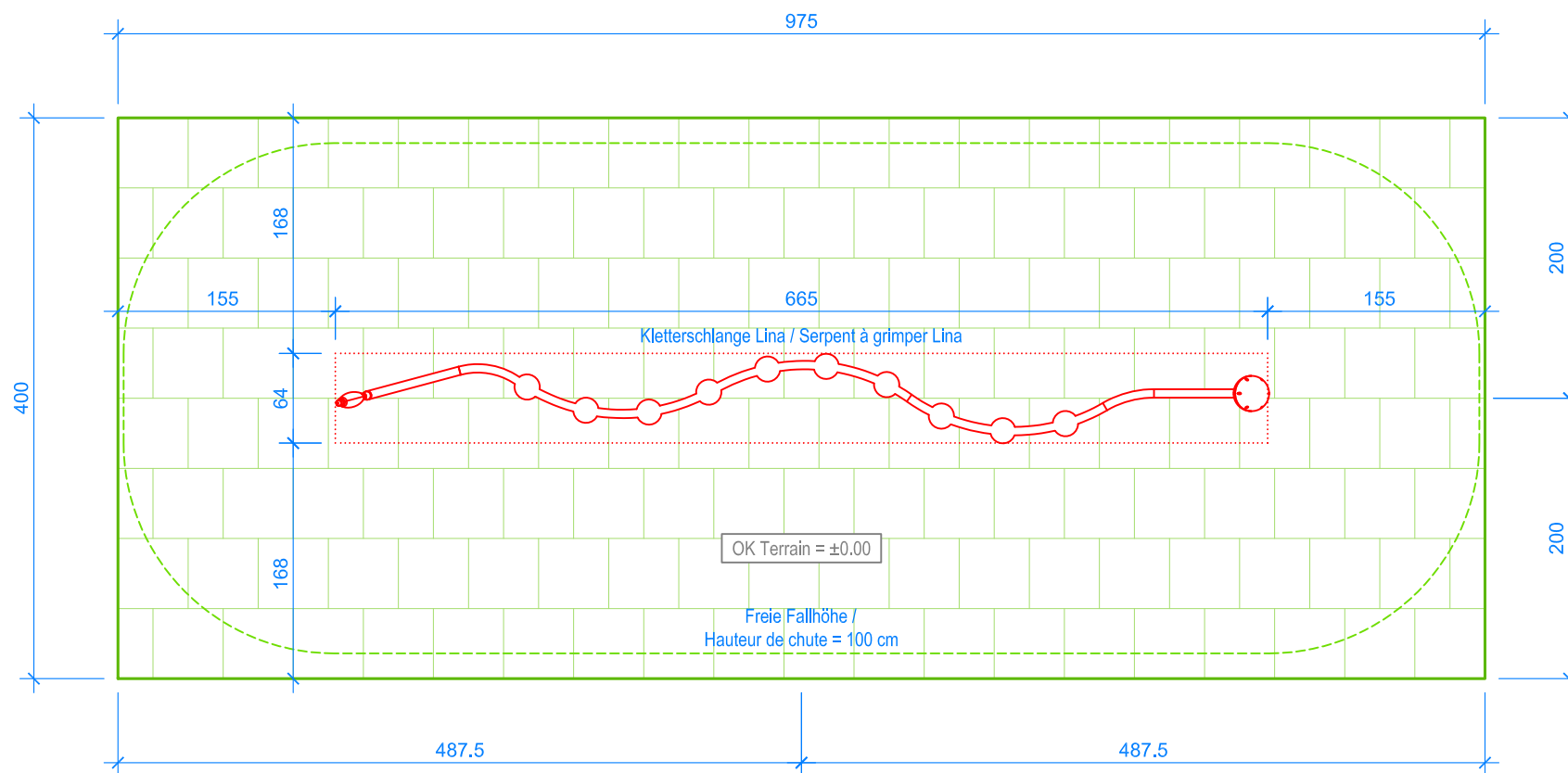
GRUNDRISS / PLAN 1:50
