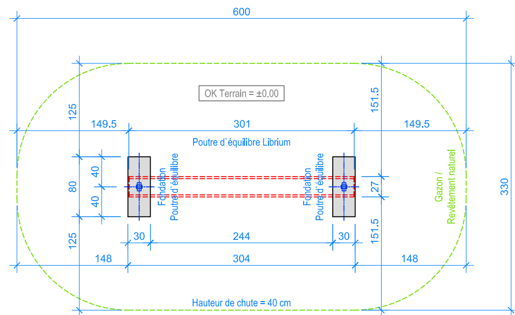
PLAN 1:50
