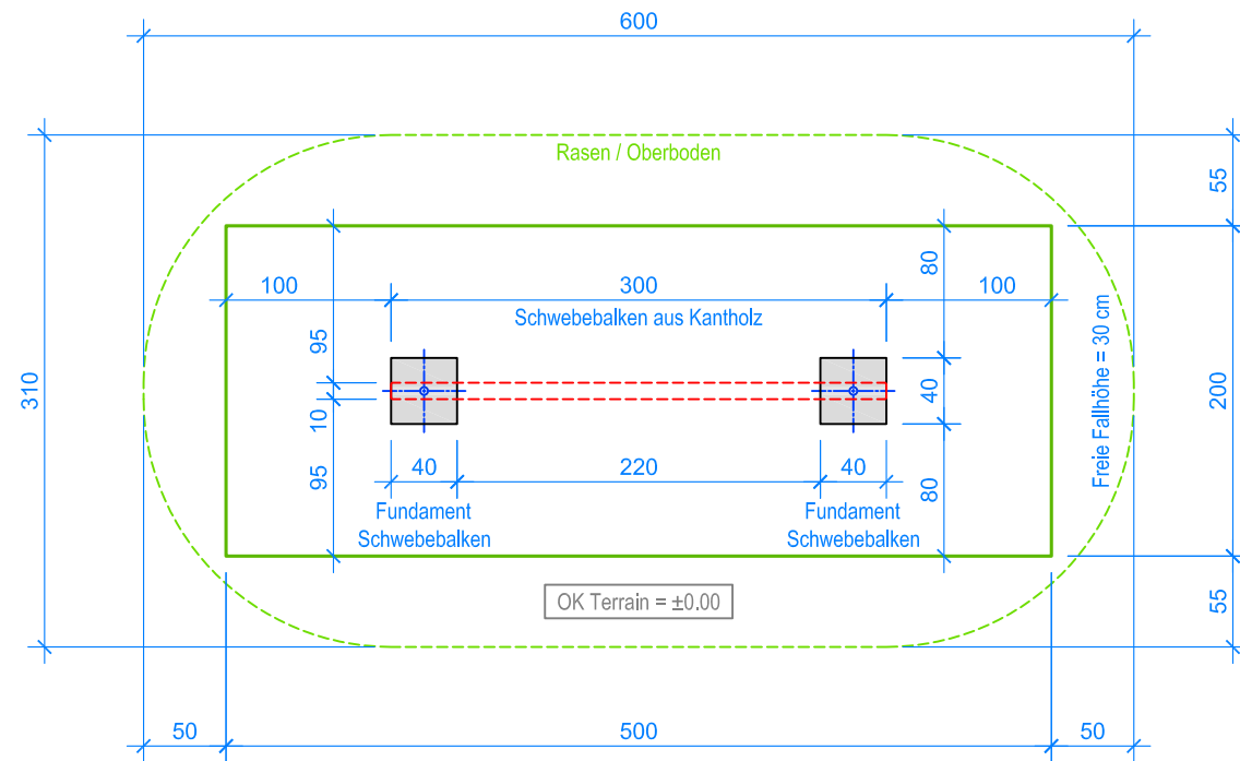
GRUNDRISS 1:50
