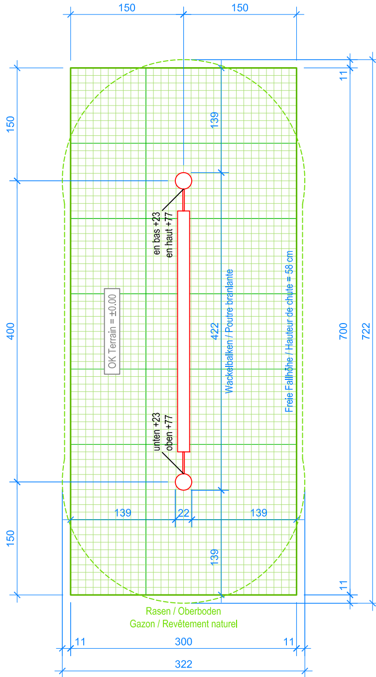
GRUNDRISS / PLAN 1:50
