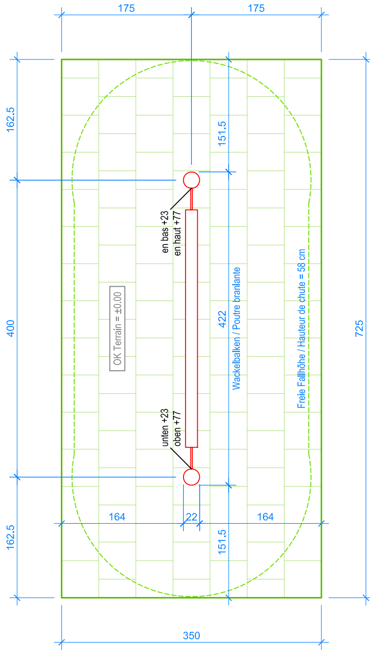
GRUNDRISS / PLAN 1:50
