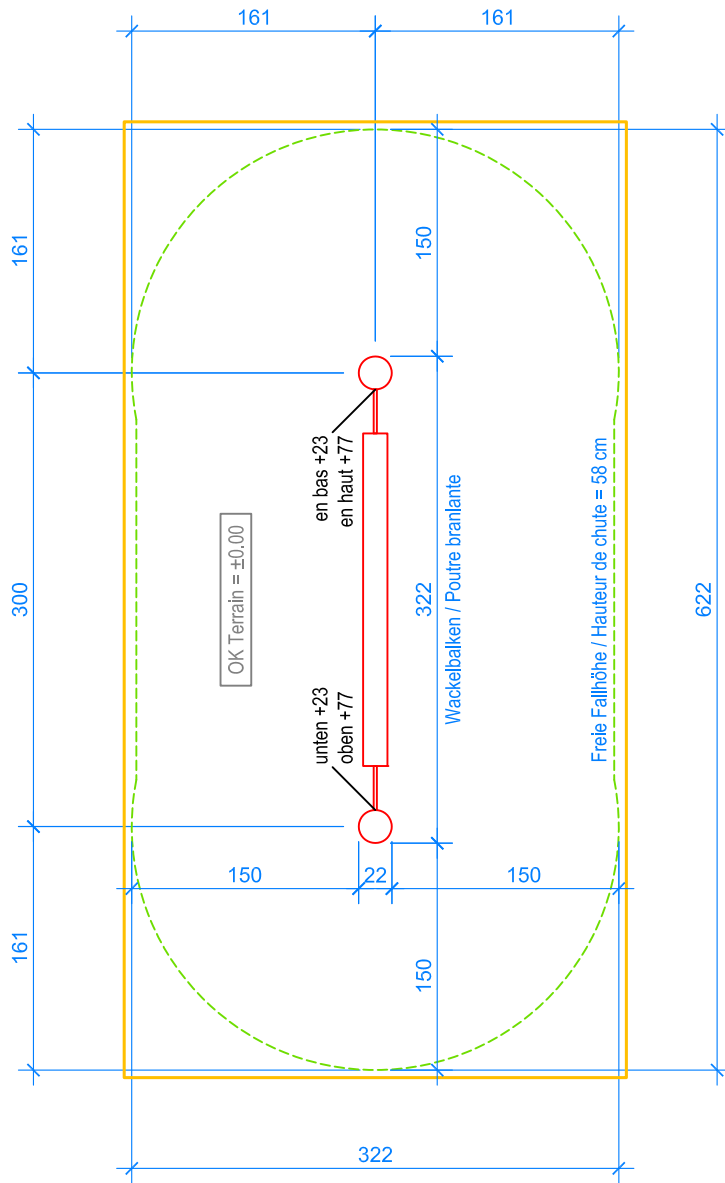
GRUNDRISS / PLAN 1:50
