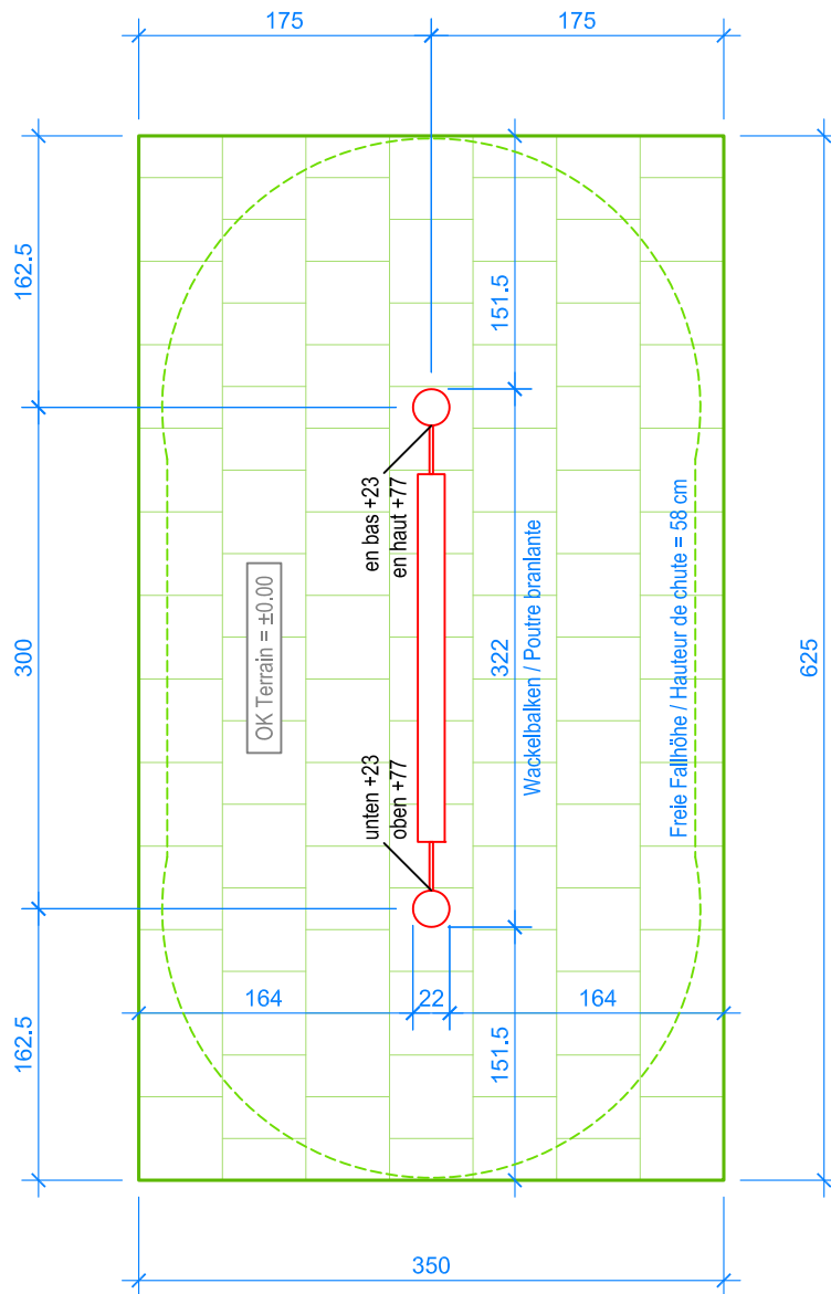
GRUNDRISS / PLAN 1:50
