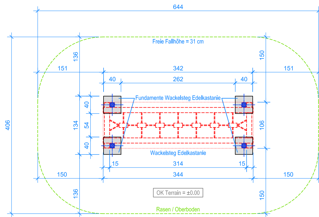
GRUNDRISS 1:50
