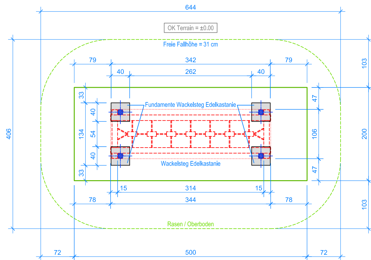
GRUNDRISS 1:50
