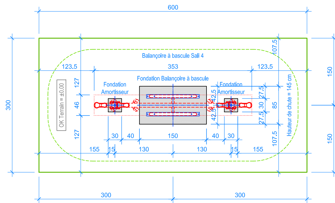
PLAN 1:50
