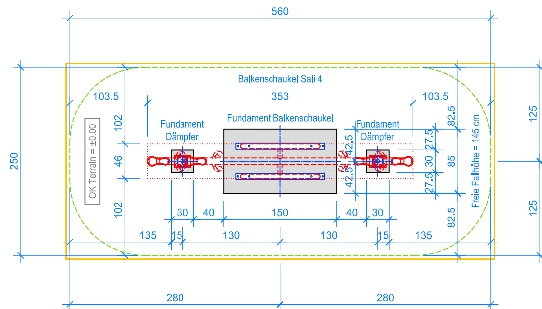
GRUNDRISS 1:50
