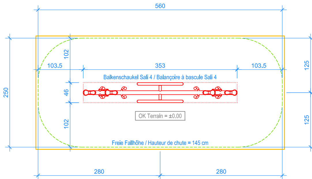
GRUNDRISS / PLAN 1:50
