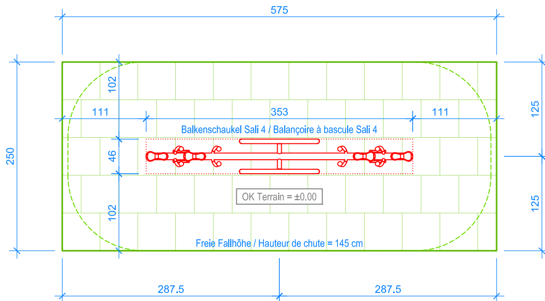
GRUNDRISS / PLAN 1:50
