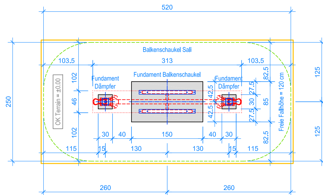
GRUNDRISS 1:50
