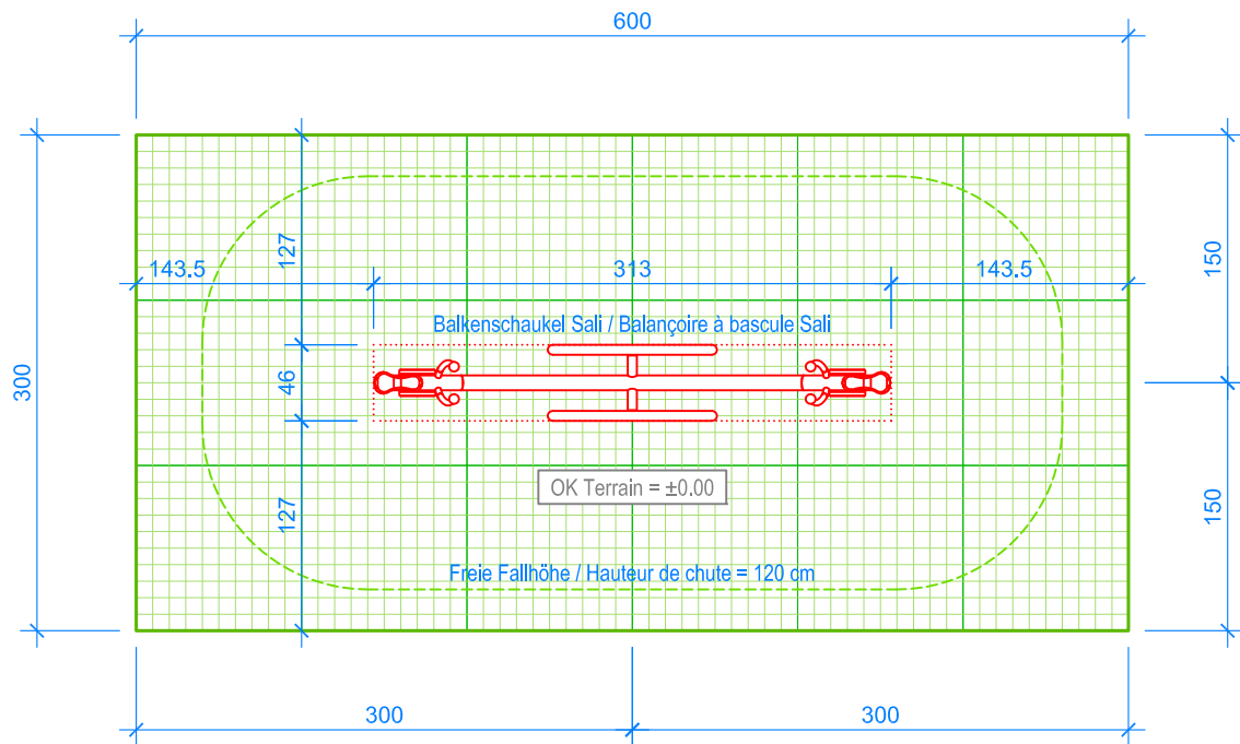
GRUNDRISS / PLAN 1:50
