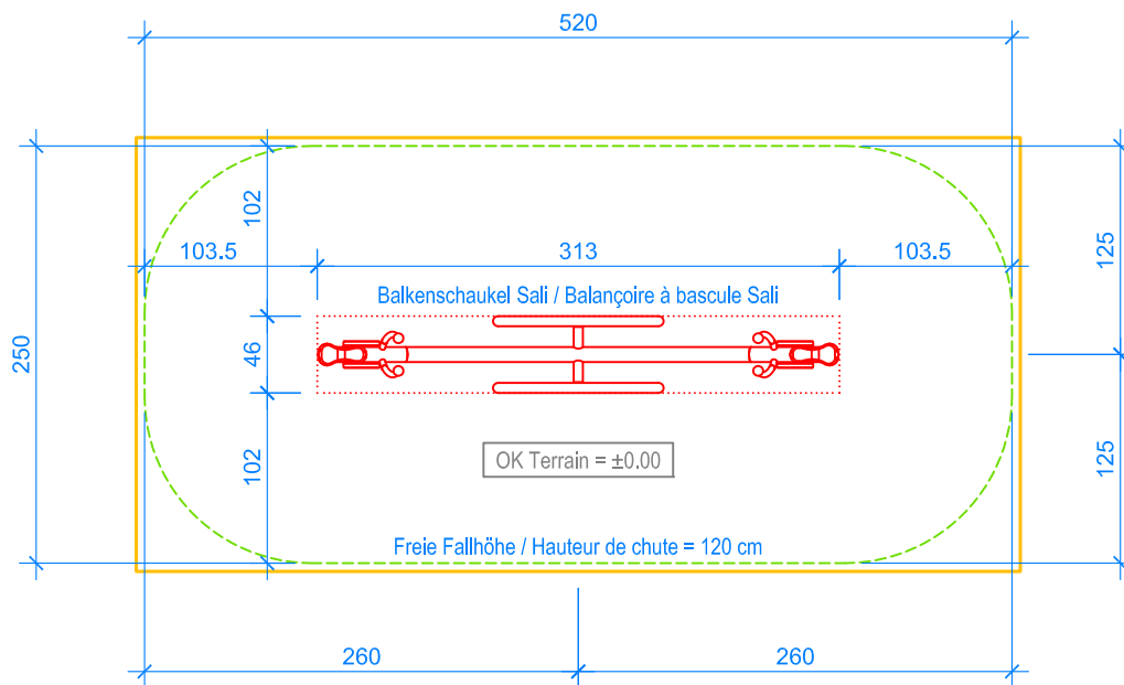
GRUNDRISS / PLAN 1:50
