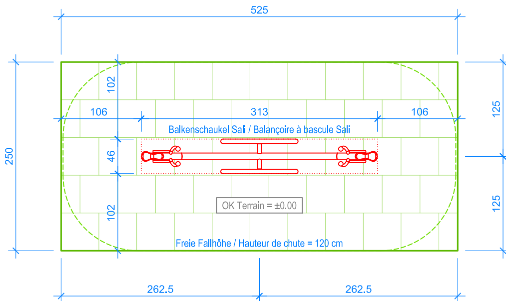
GRUNDRISS / PLAN 1:50
