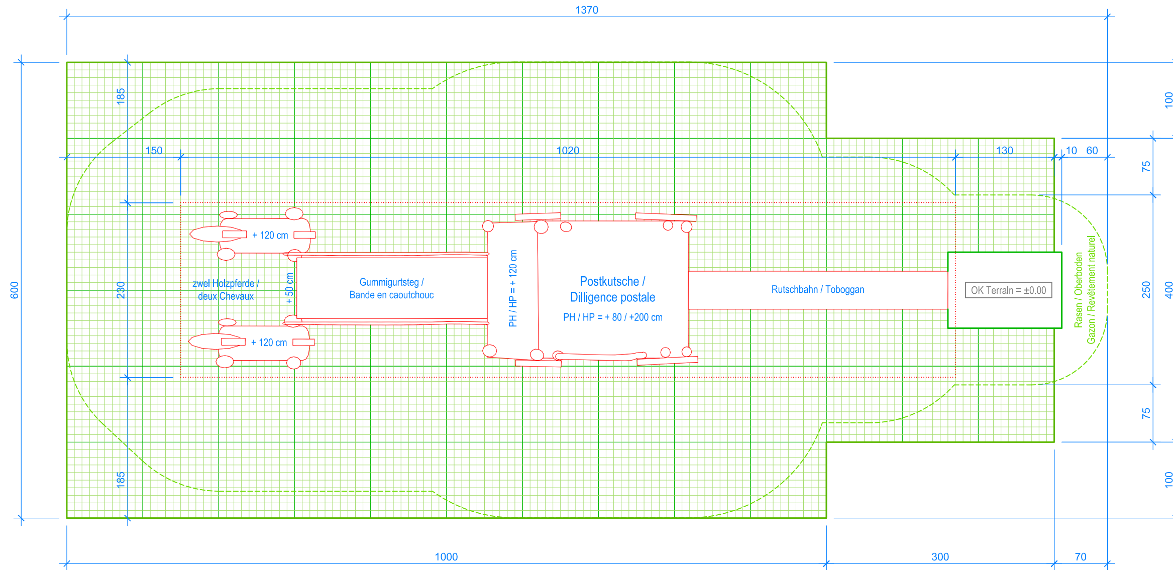
GRUNDRISS / PLAN 1:50
