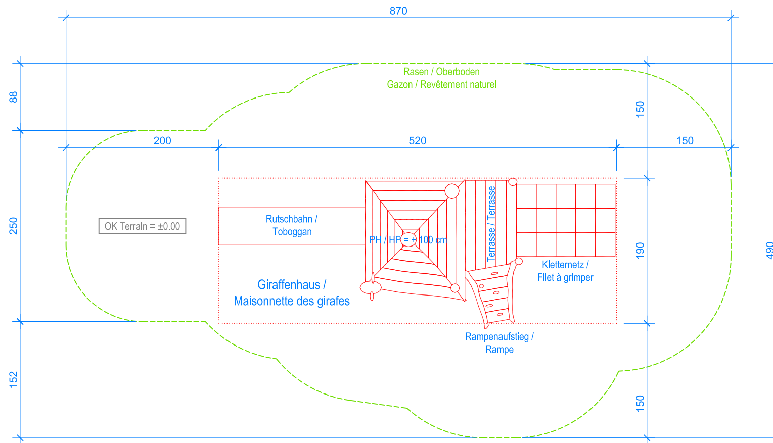
GRUNDRISS / PLAN 1:50
