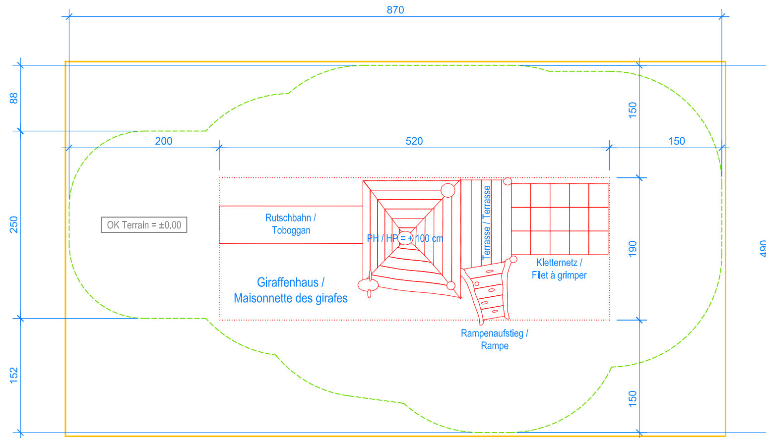
GRUNDRISS / PLAN 1:50
