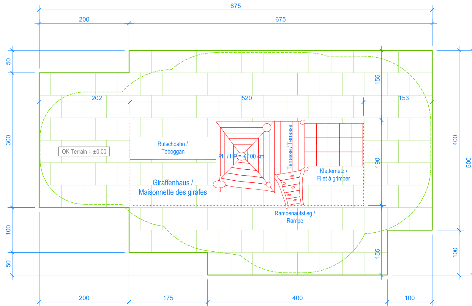
GRUNDRISS / PLAN 1:50
