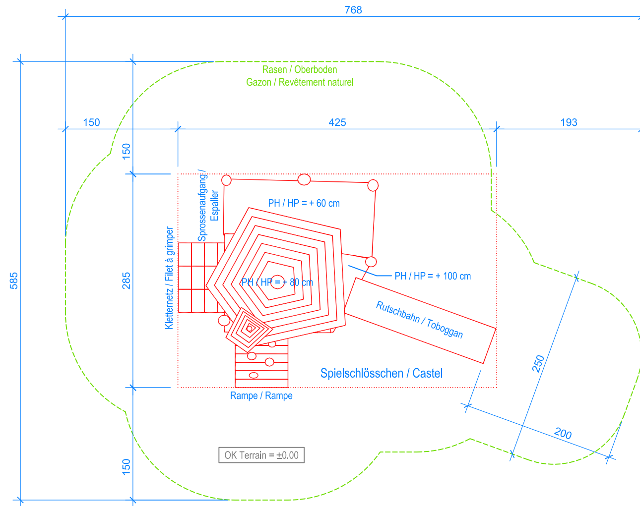
GRUNDRISS / PLAN 1:50
