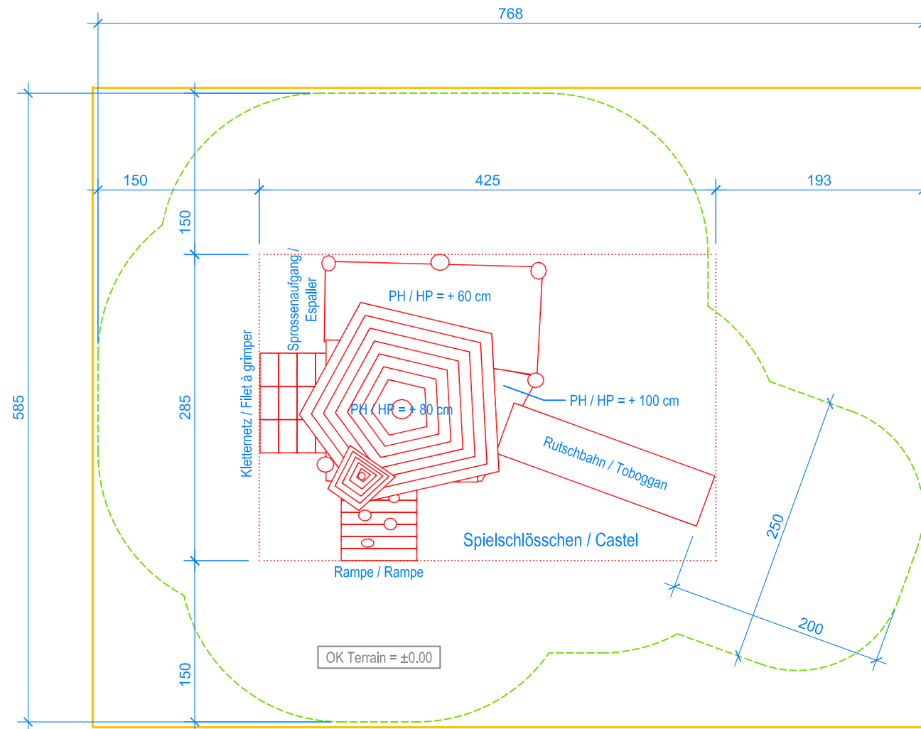
GRUNDRISS / PLAN 1:50
