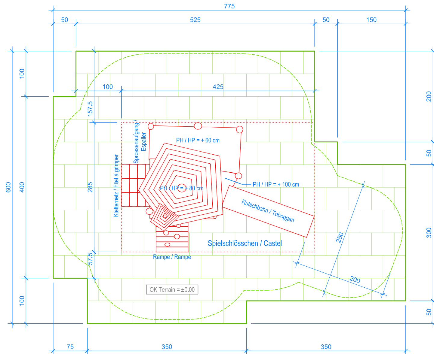
GRUNDRISS / PLAN 1:50
