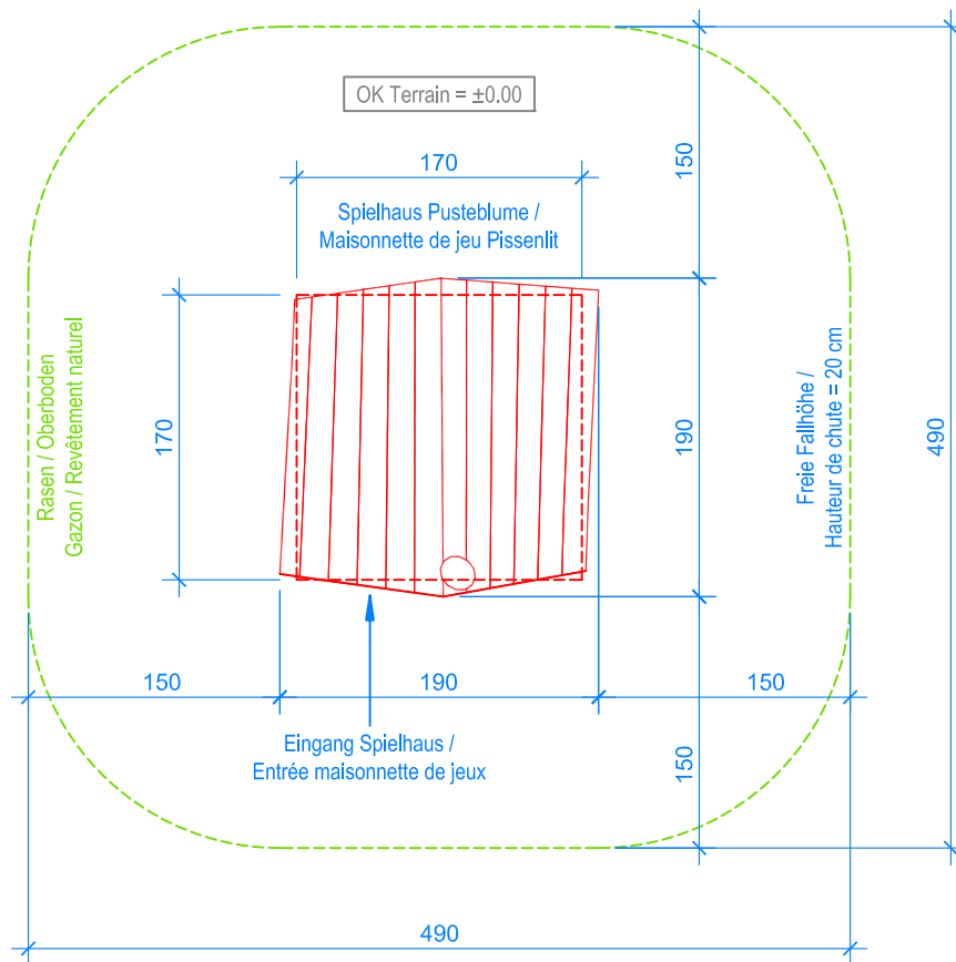
GRUNDRISS / PLAN 1:50
