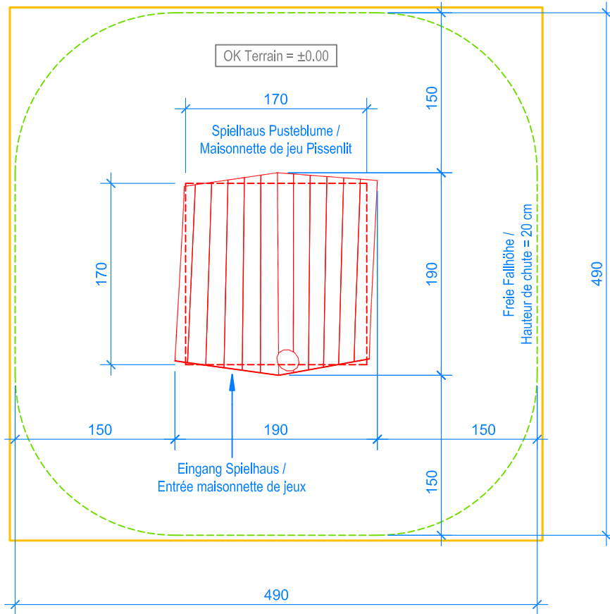
GRUNDRISS / PLAN 1:50
