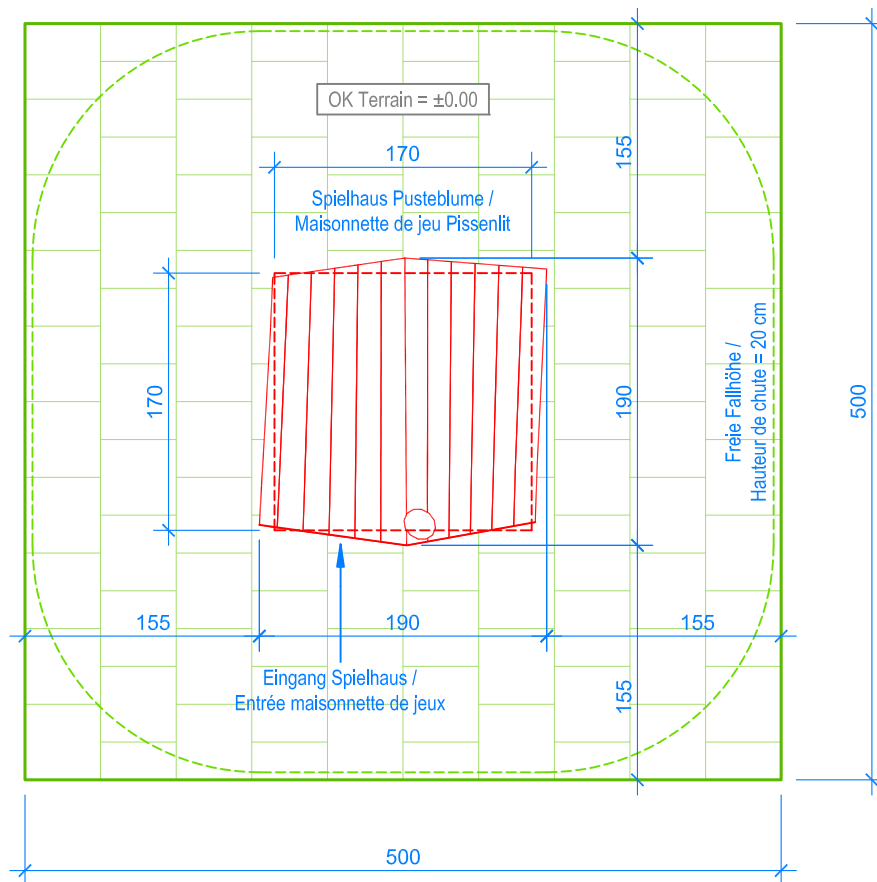
GRUNDRISS / PLAN 1:50
