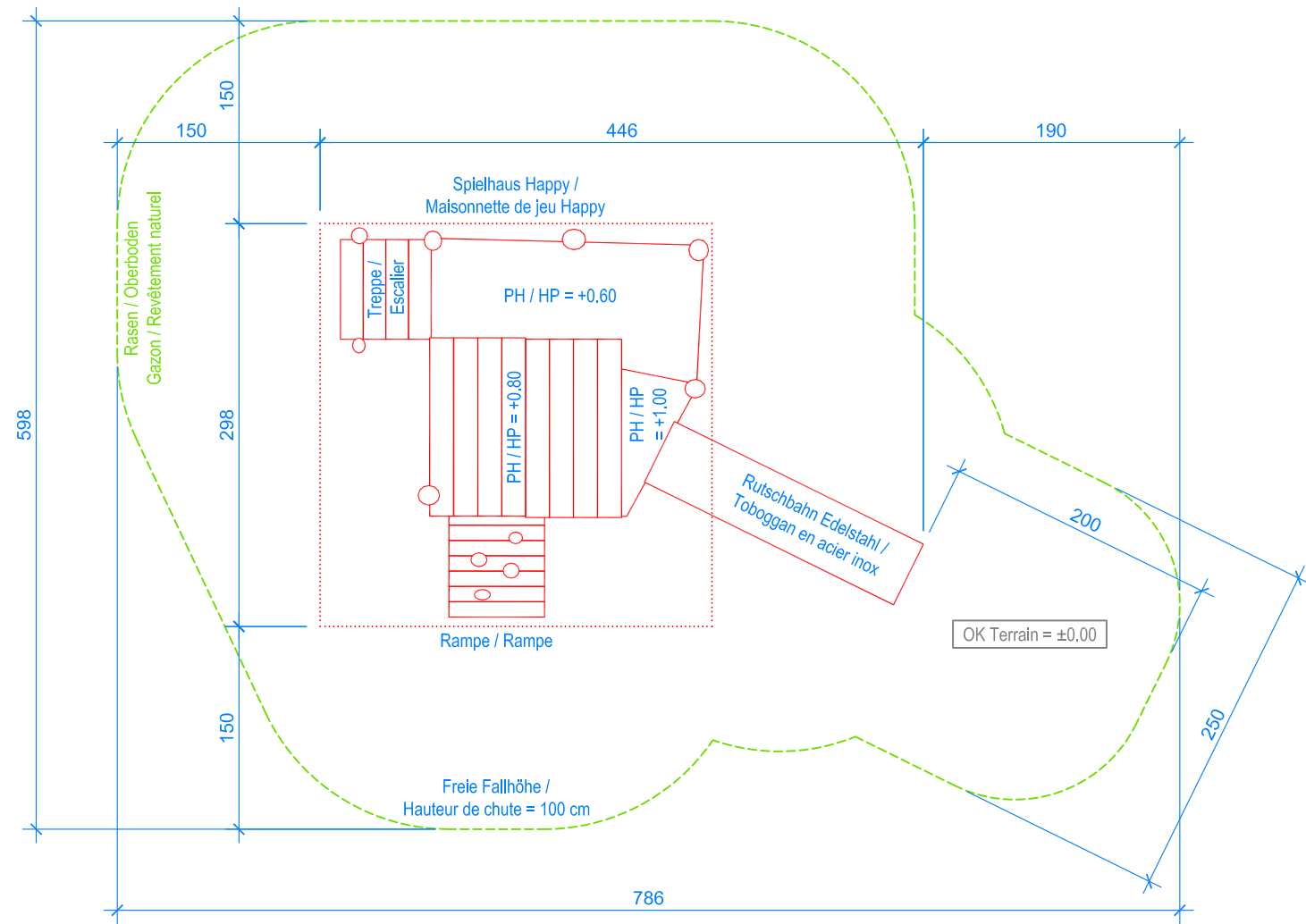
GRUNDRISS / PLAN 1:50
