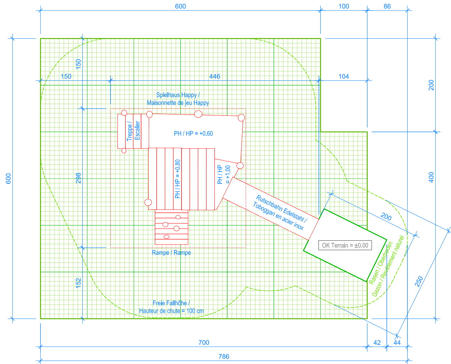
GRUNDRISS / PLAN 1:50
