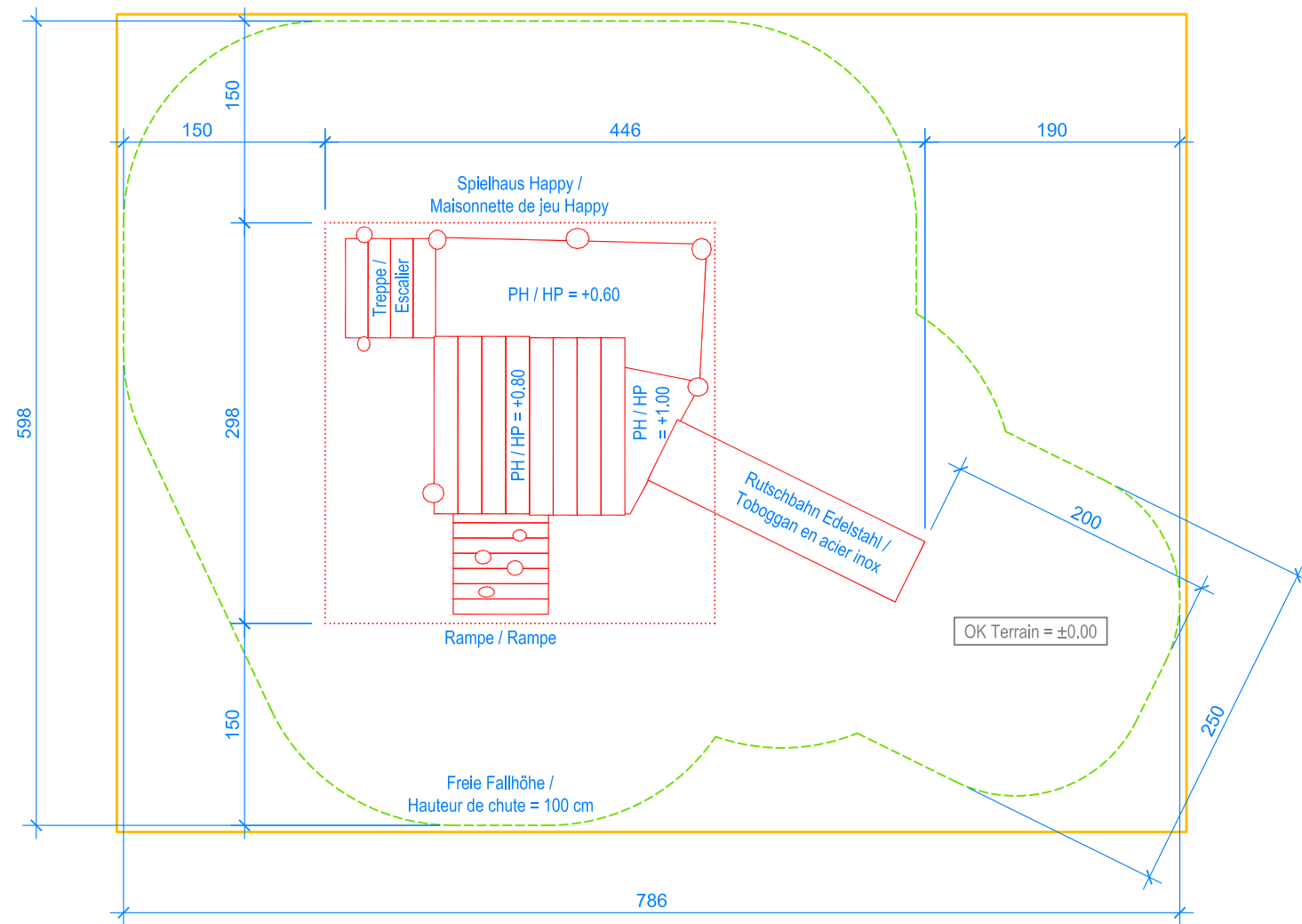
GRUNDRISS / PLAN 1:50
