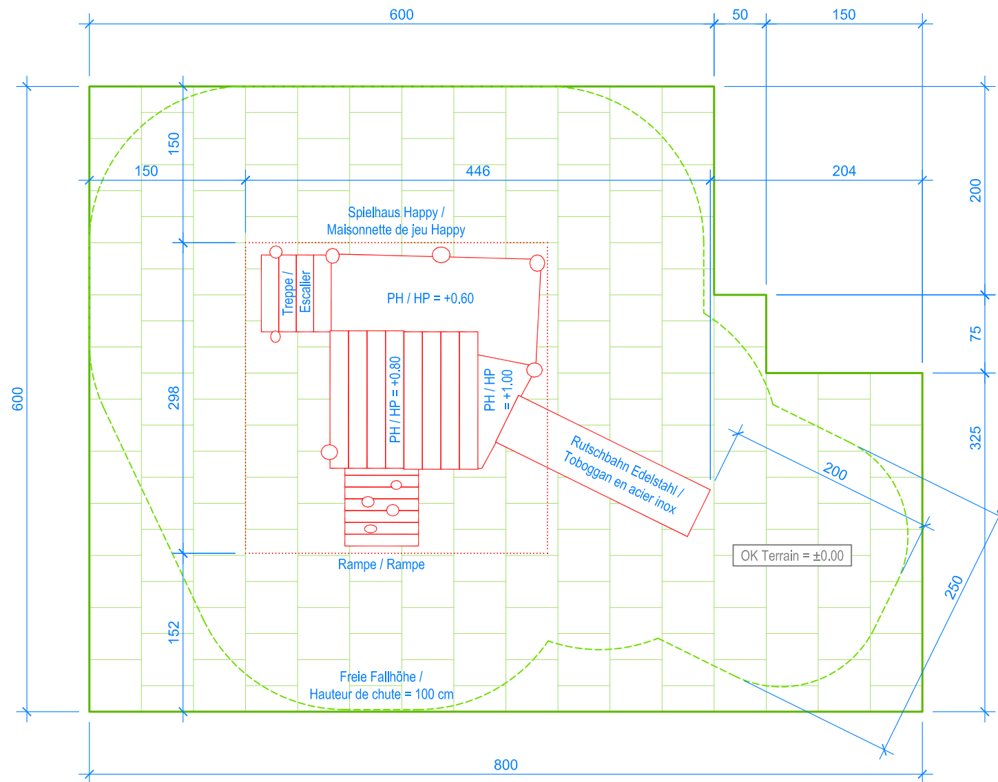
GRUNDRISS / PLAN 1:50
