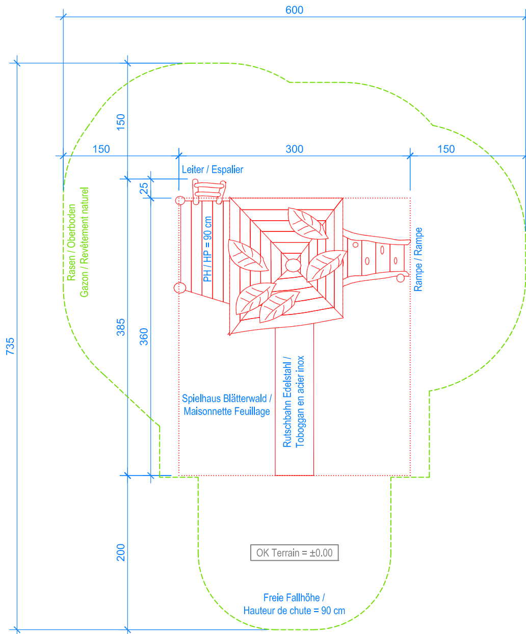
GRUNDRISS / PLAN 1:50
