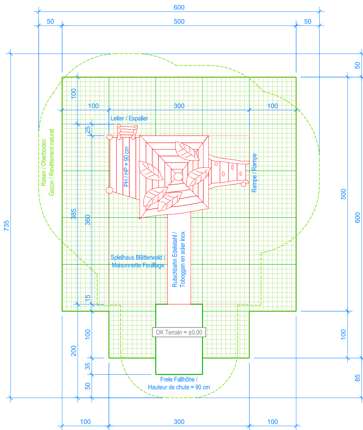
GRUNDRISS / PLAN 1:50
