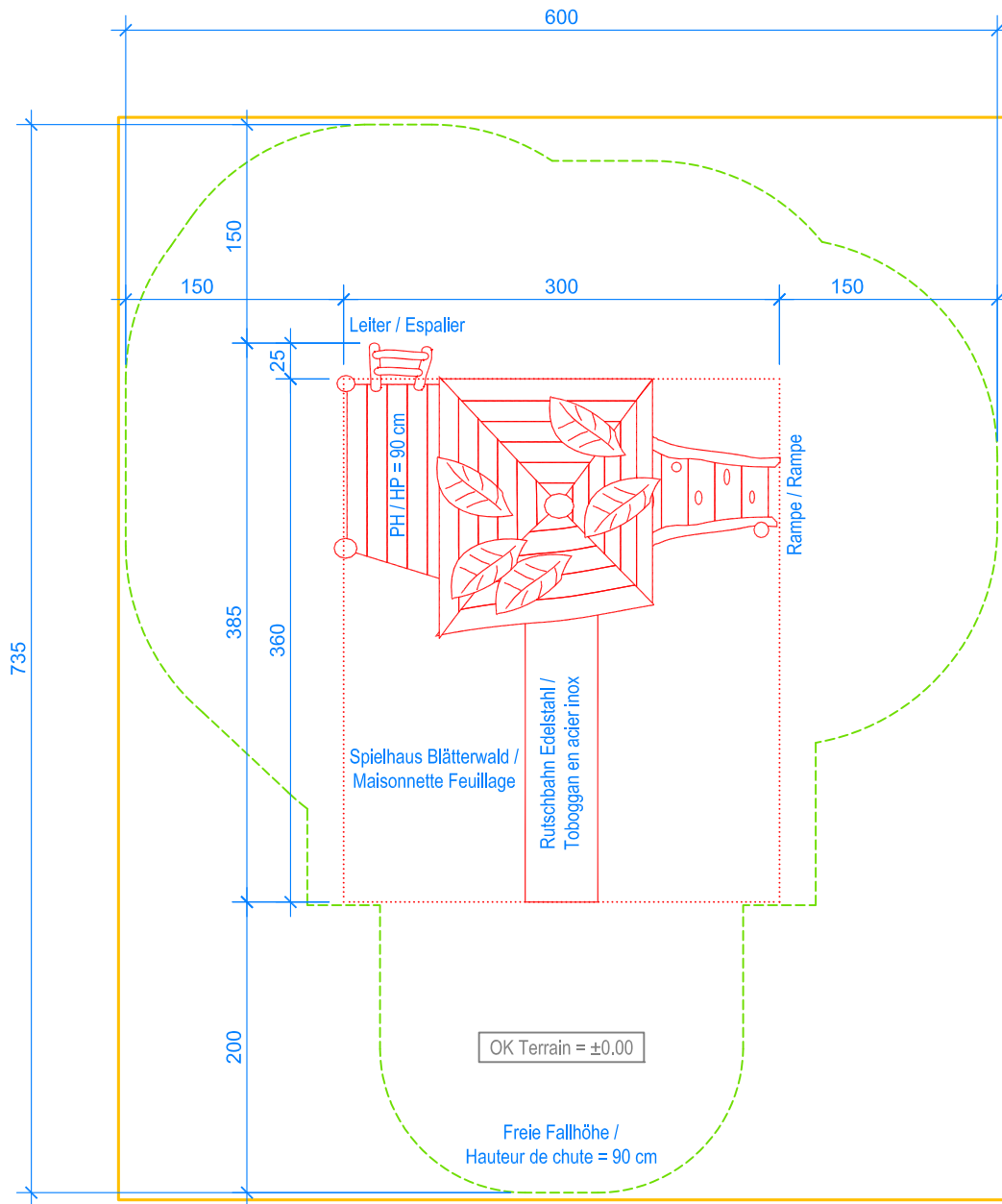
GRUNDRISS / PLAN 1:50
