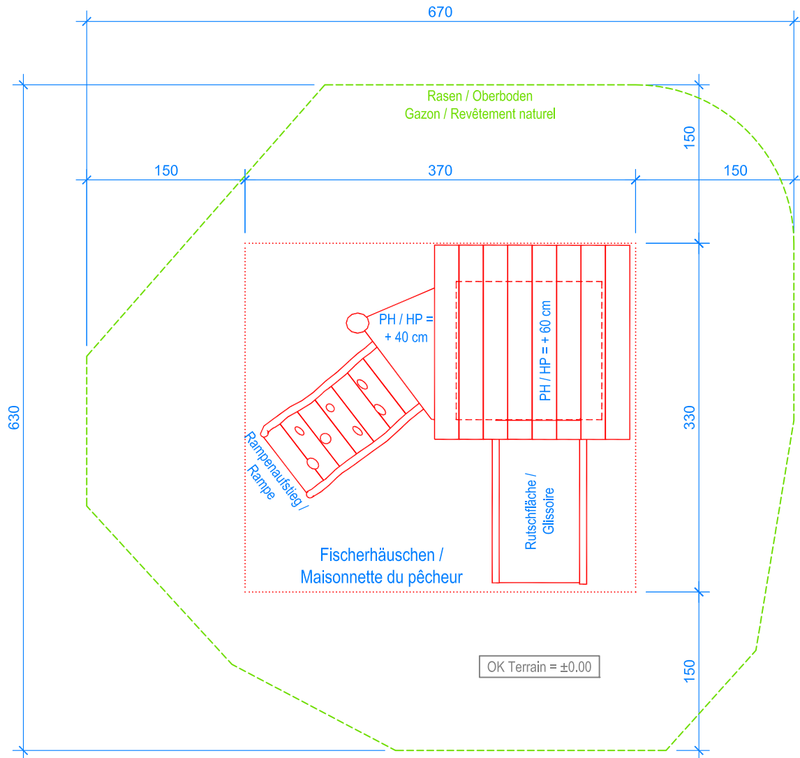
GRUNDRISS / PLAN 1:50
