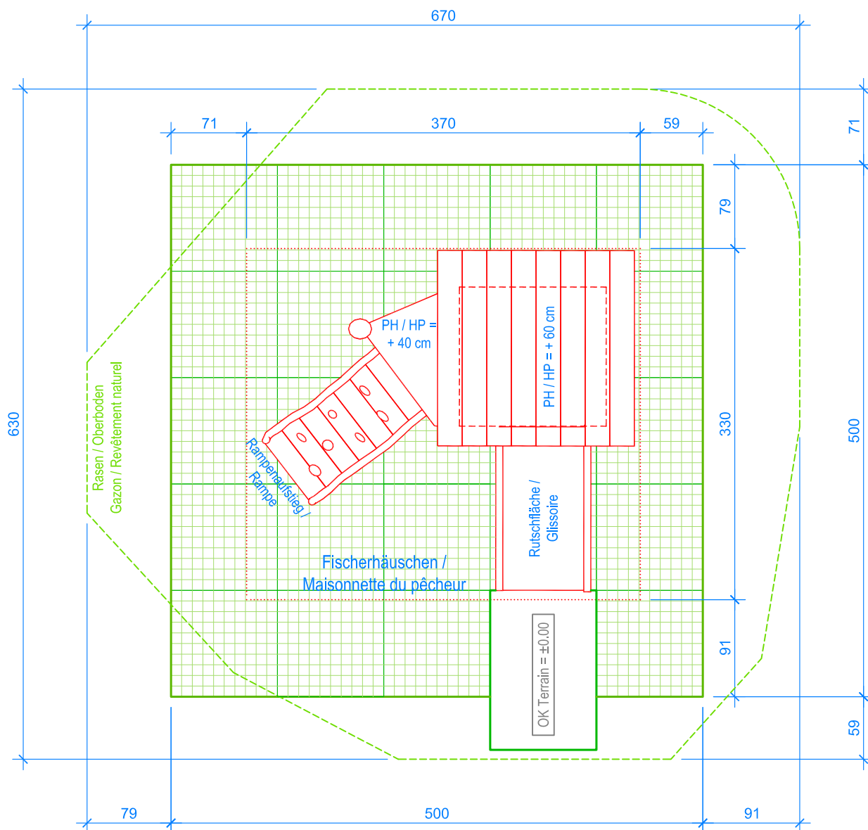
GRUNDRISS / PLAN 1:50
