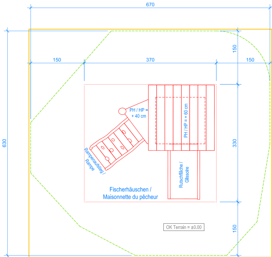
GRUNDRISS / PLAN 1:50
