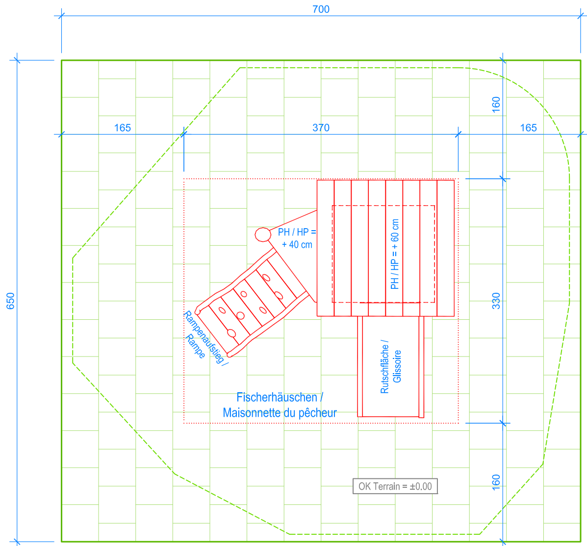
GRUNDRISS / PLAN 1:50
