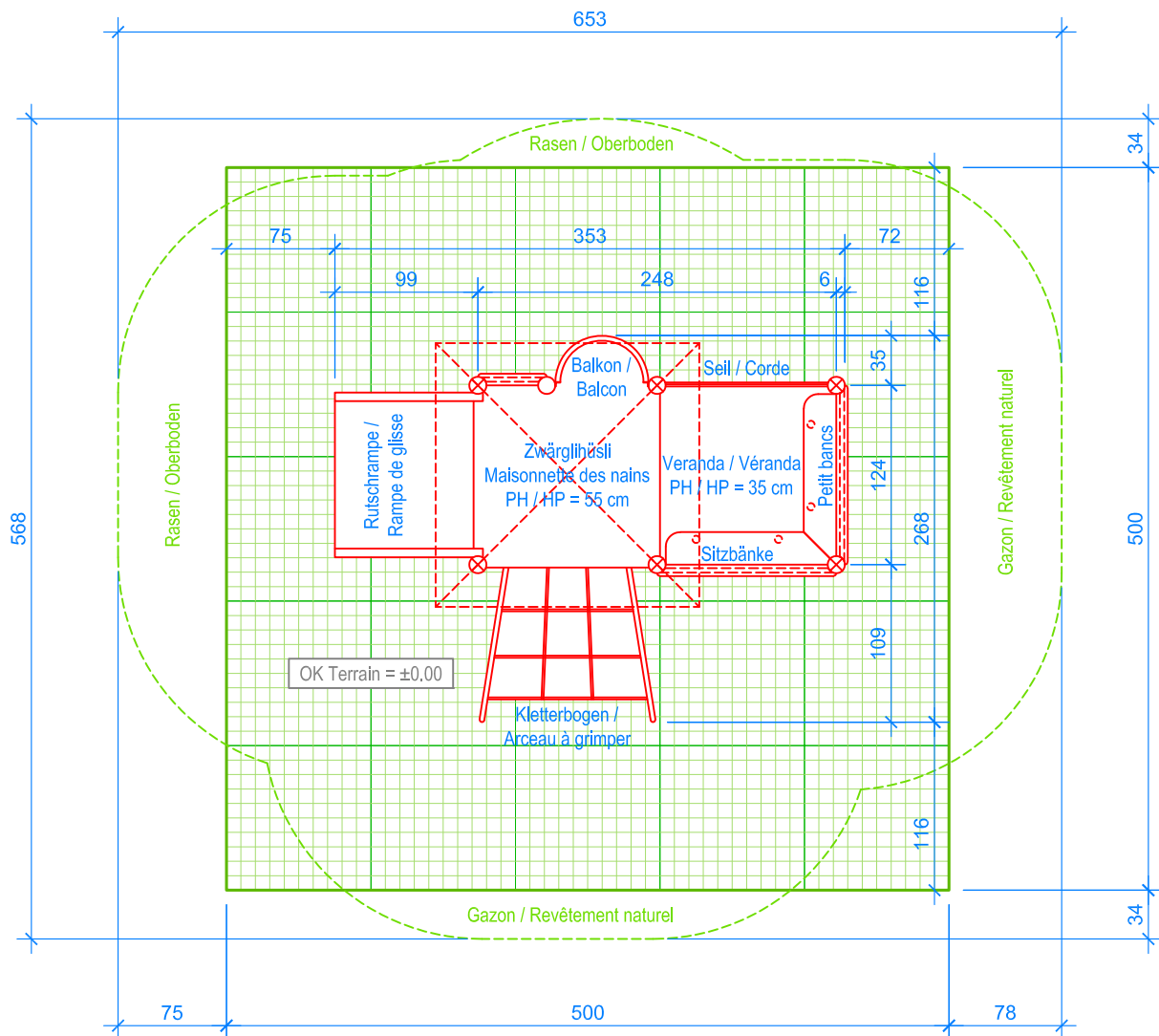
GRUNDRISS / PLAN 1:50
