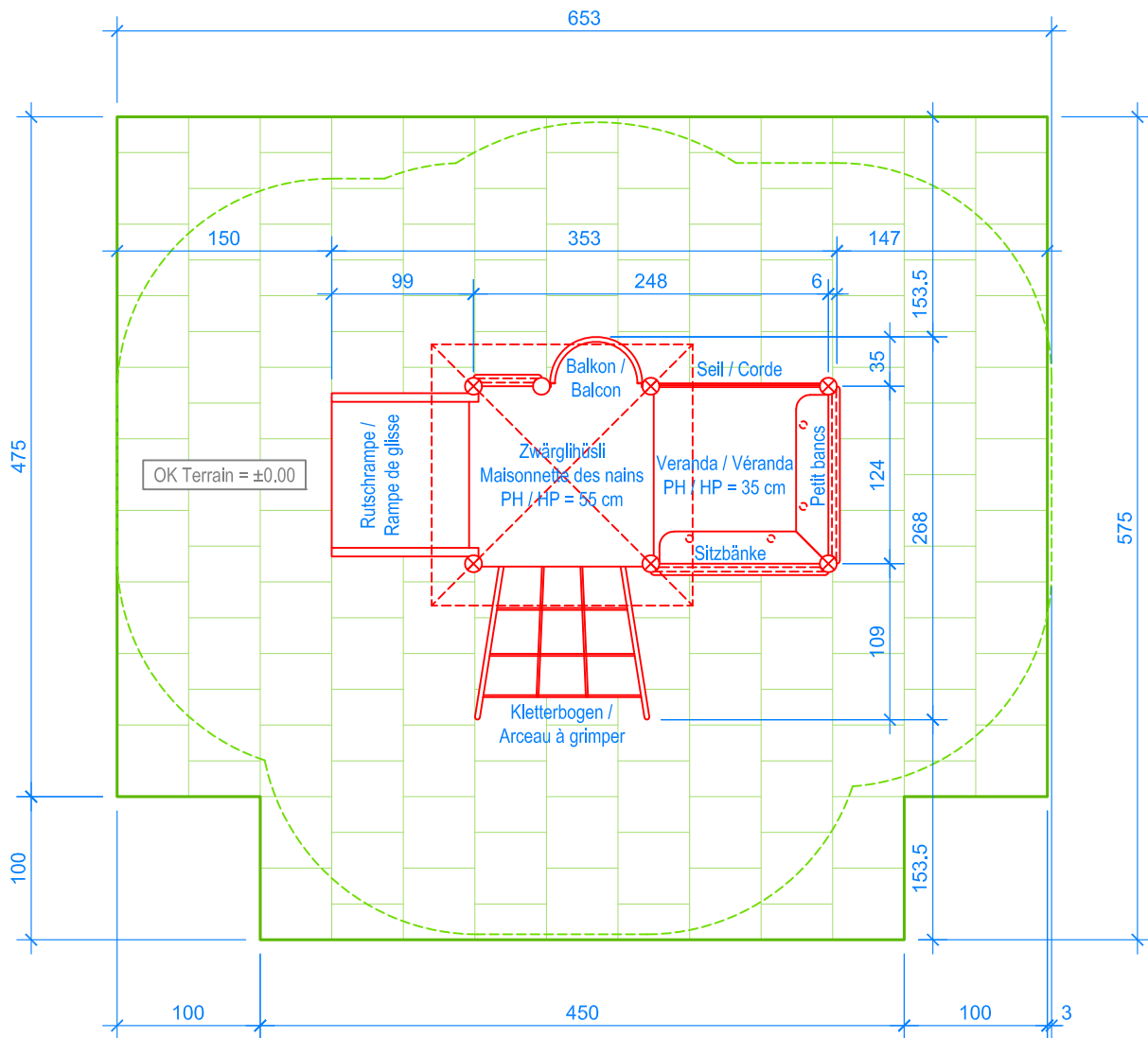
GRUNDRISS / PLAN 1:50
